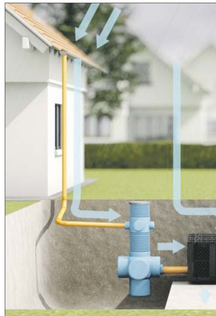
Zagospodarowanie wody deszczowej – skrzynki rozsączające
